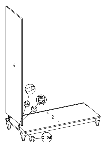
③ Alt parçaya sol yan parça montajı
